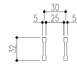
ベアリングバー 詳細図
