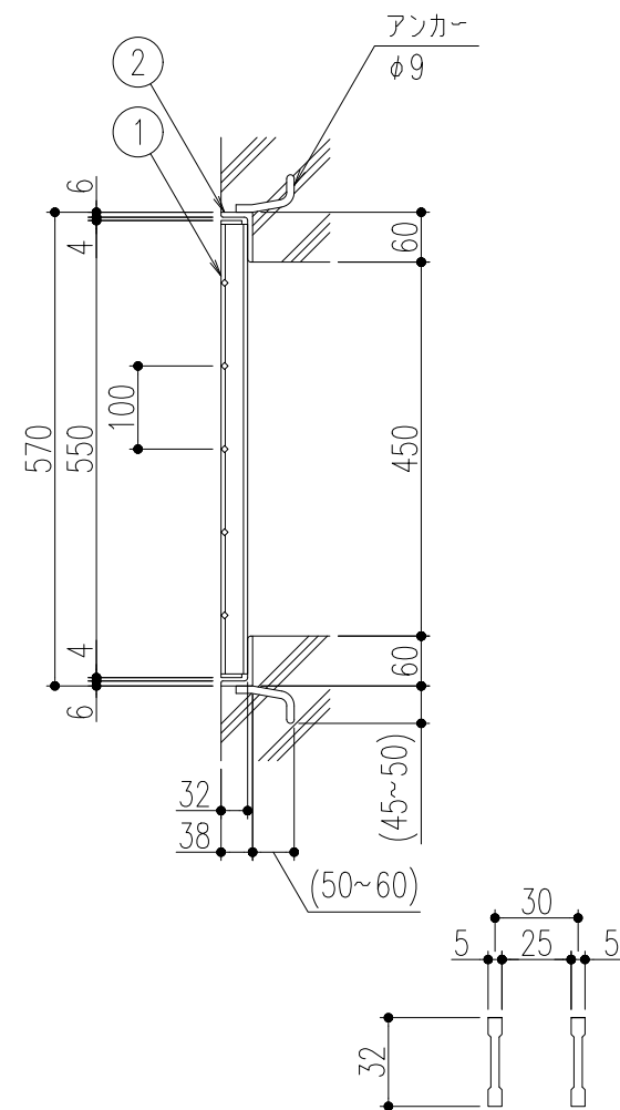
2 受枠 8.9 kg/本 SS400 錆止め塗装(黒) ベアリングバー 詳細図 1 蓋 21.2 kg/枚 SS400 溶融亜鉛めっき 品番 名称 質量 材質 表面処理 備考 △ 第三 角 法 製 図 朱 検 図 胡 承 認 後 藤 担 当 年 月 日 尺 度 名 称 側溝用スチールグレーチング 図 番 SSAAAI0045 △ △ 記 号 変更内容・理由 年 月 日 担 当 承 認 品 名 蓋 : CB32-4.5 受枠 : GT-1-32 株式会社 中部コーポレーション
