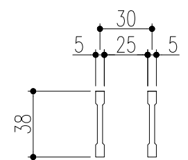
ベアリングバー 詳細図
