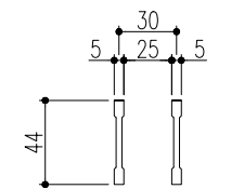
ベアリングバー 詳細図
