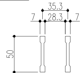
ベアリングバー 詳細図
