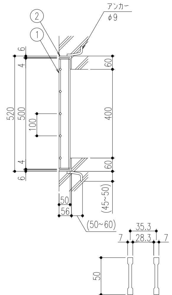
ベアリングバー 詳細図
