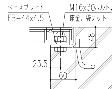
ボルト固定部詳細図 (S=1/5)
