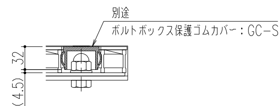
ゴムカバー装着図 (S=1/5)
