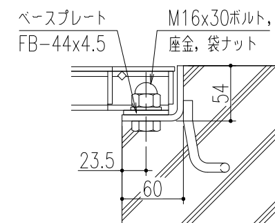
ボルト固定部詳細図 (S=1/5)
