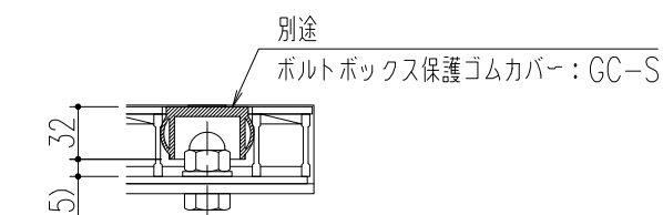
ゴムカバー装着図 (S=1/5)
