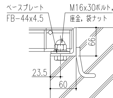
ボルト固定部詳細図 (S=1/5)
