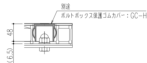
ゴムカバー装着図 (S=1/5)
