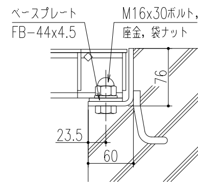
ボルト固定部詳細図 (S=1/5)
