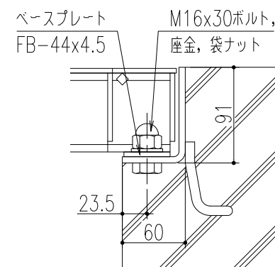
ボルト固定部詳細図 (S=1/5)
