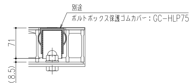
ゴムカバー装着図 (S=1/5)
