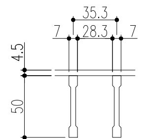
ベアリングバー 詳細図
