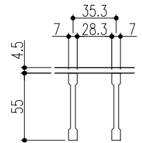
ベアリングバー 詳細図
