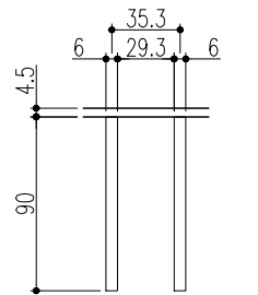
ベアリングバー 詳細図
