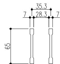
ベアリングバー 詳細図
