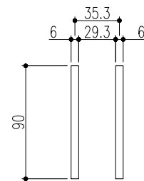
ベアリングバー 詳細図
