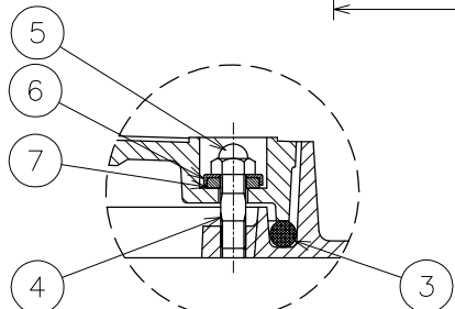
ボルト固定部詳細図
