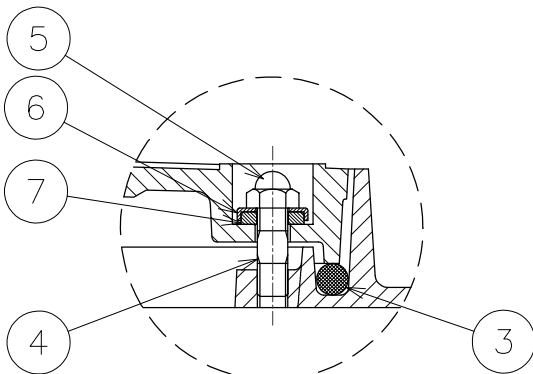
ボルト固定部詳細図
