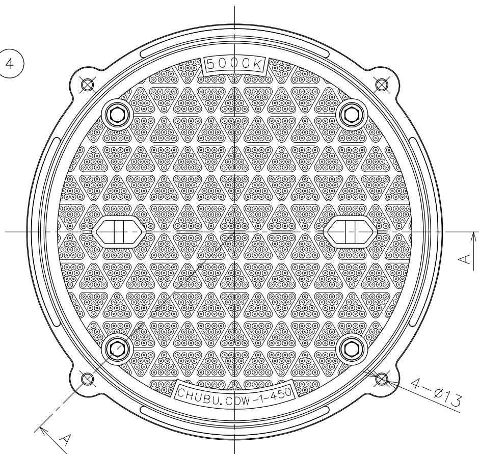
ボルト固定部詳細図 (1/3)
