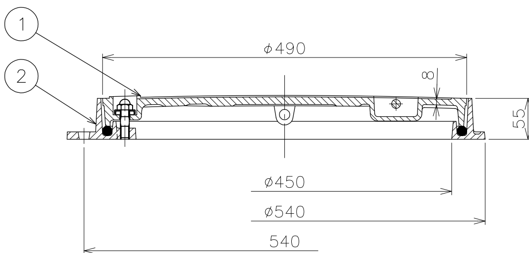
A-A断面
