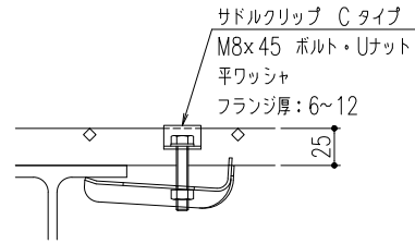
サドルクリップ Cタイプ固定 1/4
