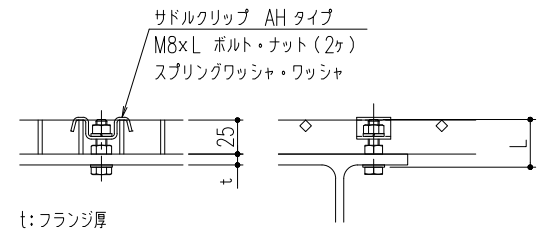
サドルクリップ AHタイプ固定 1/4
