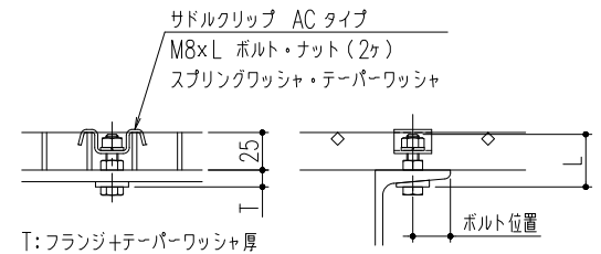
サドルクリップ ACタイプ固定 1/4
