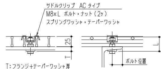
サドルクリップ ACタイプ固定 1/4
