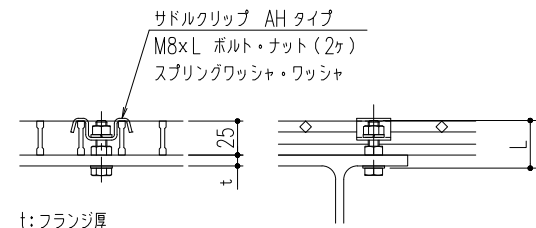
サドルクリップ AHタイプ固定 1/4
