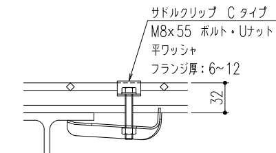
サドルクリップ Cタイプ固定 1/4
