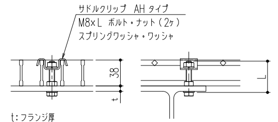
サドルクリップ AHタイプ固定 1/4
