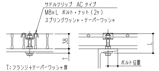
サドルクリップ ACタイプ固定 1/4
