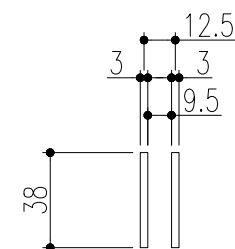
ベアリングバー 詳細図
