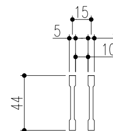
ベアリングバー 詳細図
