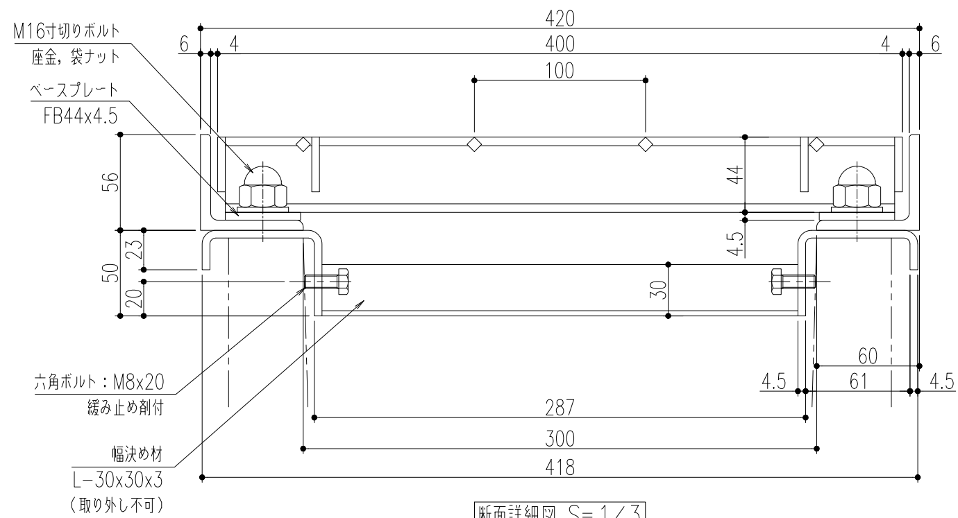
断面詳細図 S= 1/3
