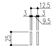
ベアリングバー 詳細図
