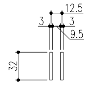
ベアリングバー 詳細図
