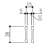
ベアリングバー 詳細図
