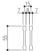
ベアリングバー 詳細図
