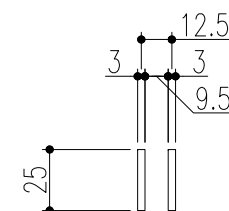
ペアリングバー 詳細図
