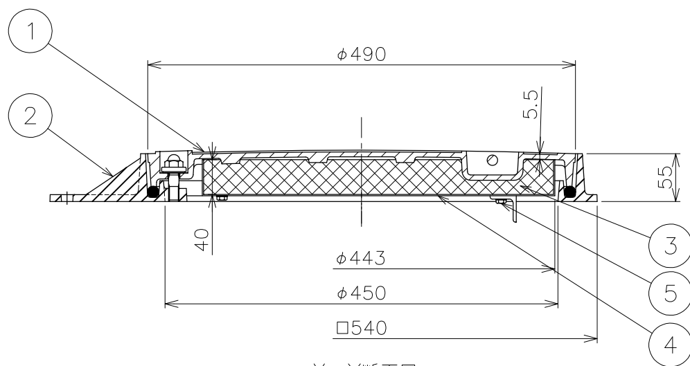
X-Y断面図
