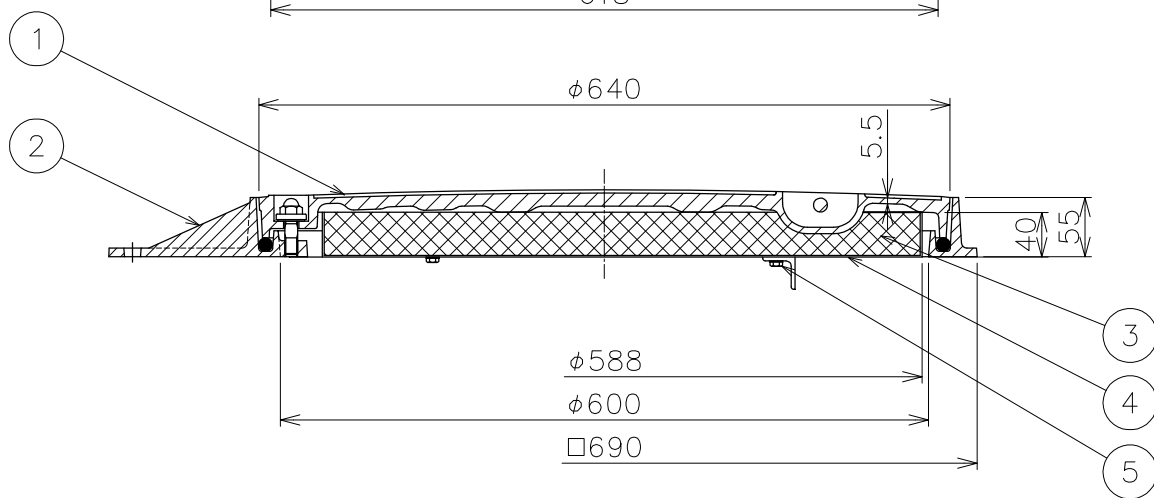
X-Y断面図
