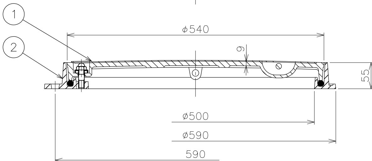
A-A断面
