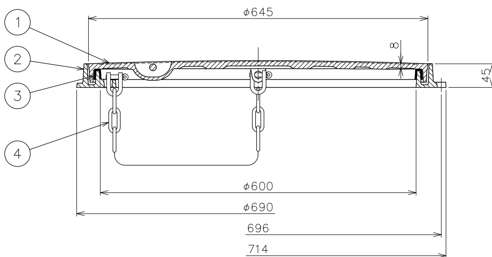
A-A断面
