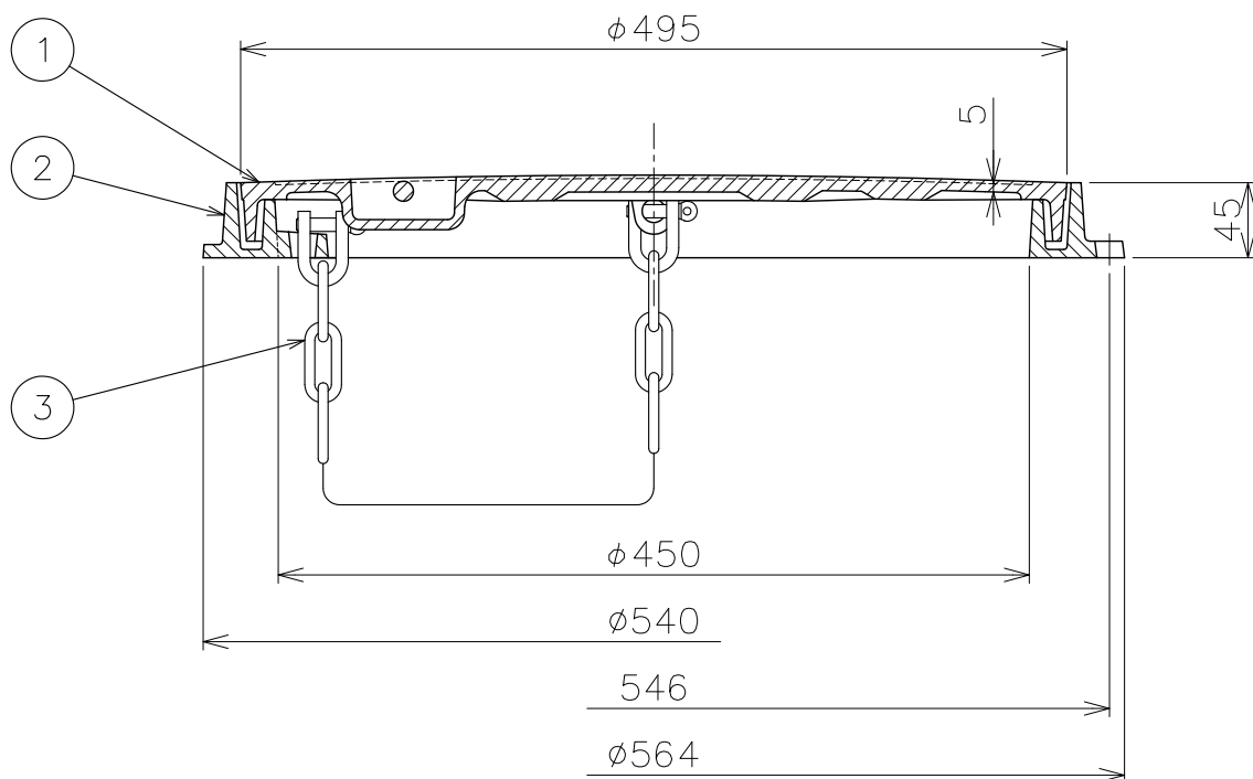
A-A断面
