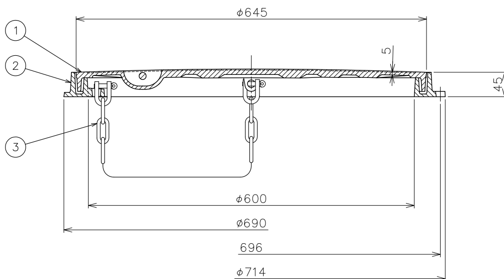
A-A断面
