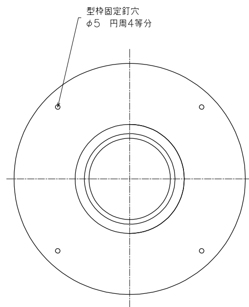
底面図
