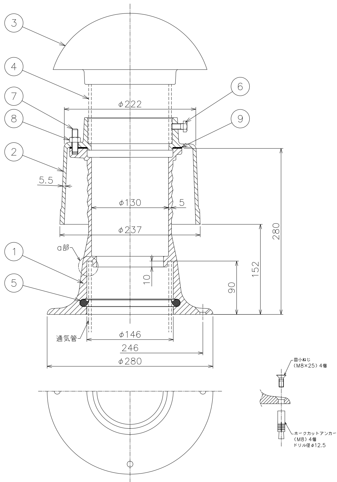
都市再生機構 型防水継手 (機械設備設計図集 J-501)
