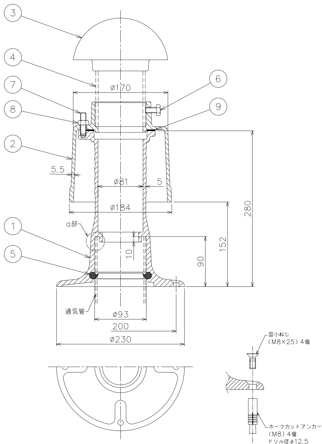
都市再生機構 型防水継手 (機械設備設計図集 J-501)
