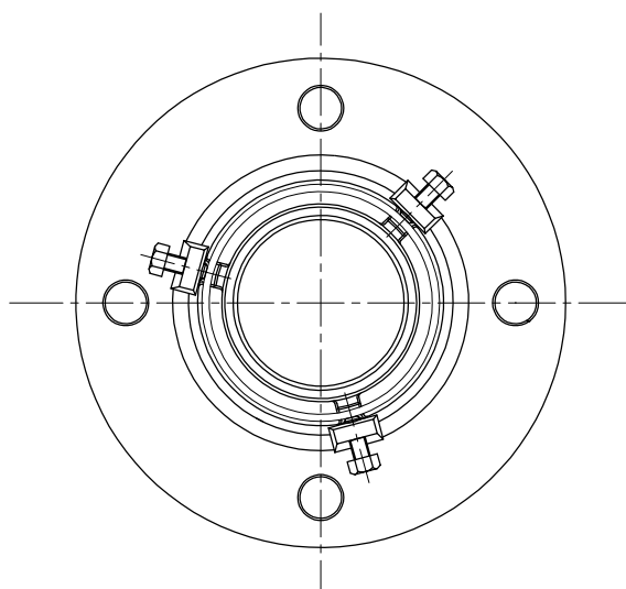
底面図
