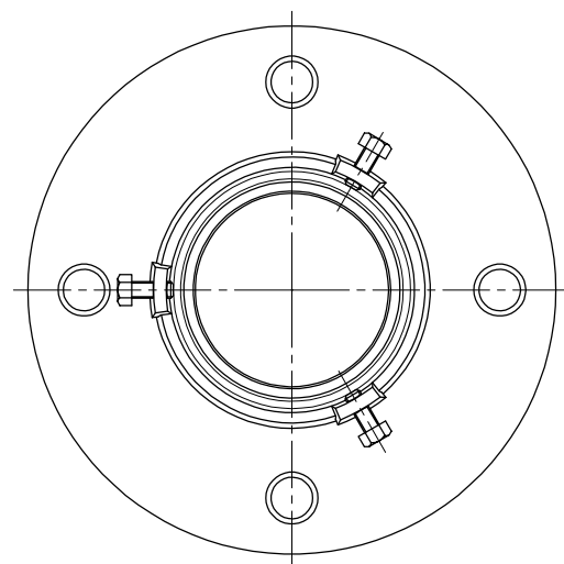
底面図
