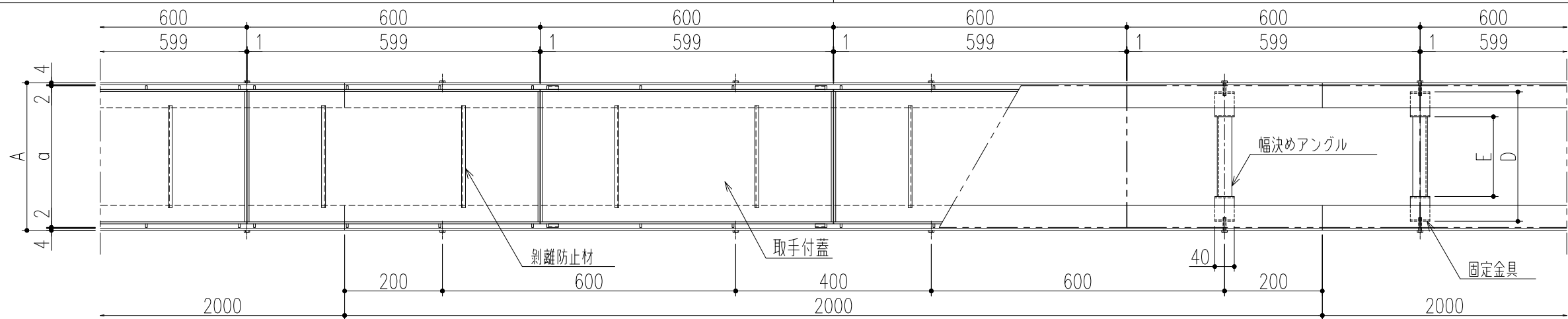
平面詳細図 S=1/10
