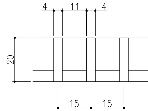
フラットバー詳細図
