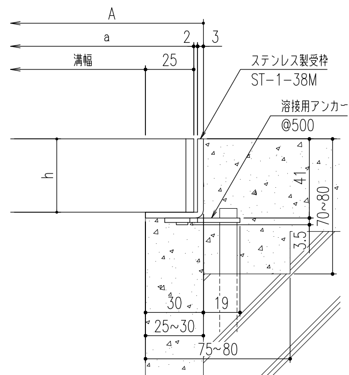
断面詳細図
