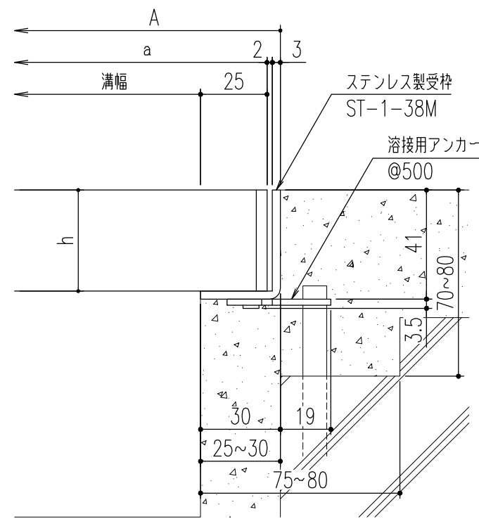
断面詳細図
