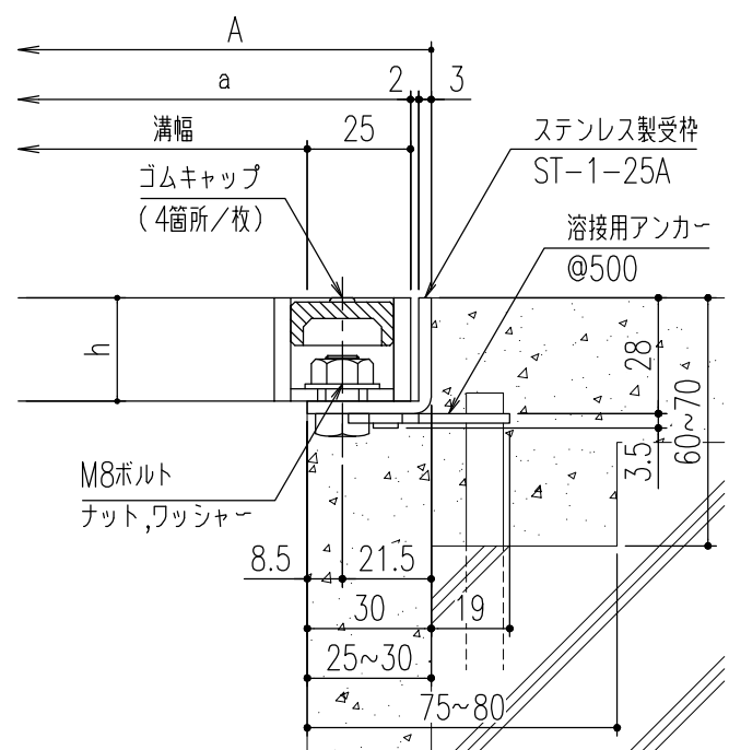
断面詳細図
