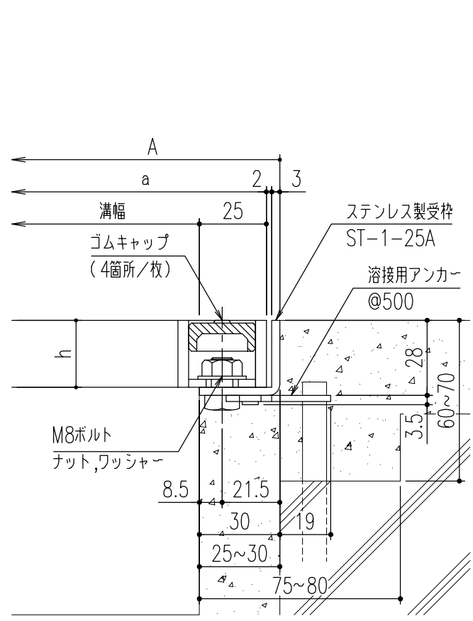
断面詳細図
