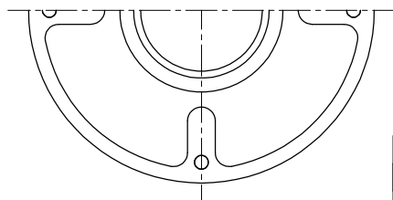
都市再生機構 型防水継手 (機械設備設計図集 J-501)
