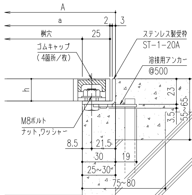
断面詳細図
