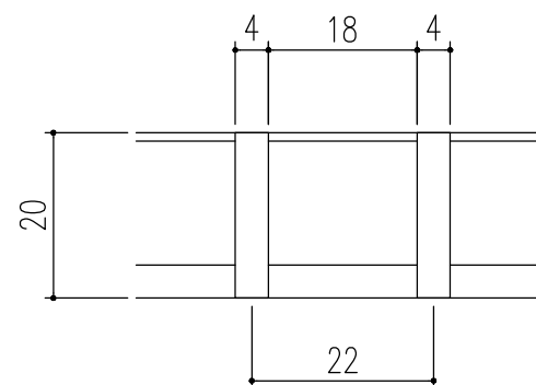
フラットバー詳細図
